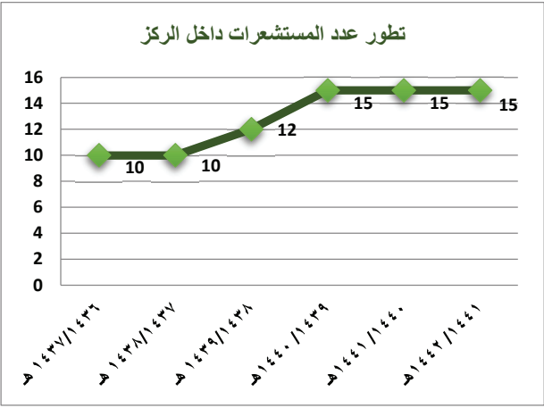
شكل (٤/٥/٢/٥) تطور عدد المستشعرات داخل المركز
